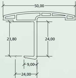
BATTUE MOULURE 50 X 9 OU 50 X 24
