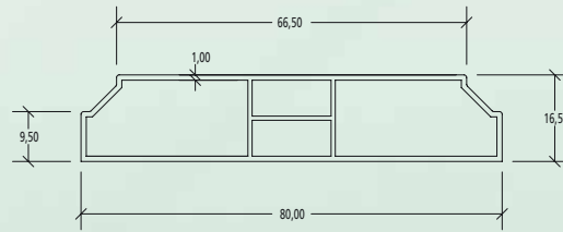
BARRE A ECHARPE
